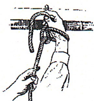
Рис. 4 «в». Закрепление спасательной веревки за конструкцию четвертым способом.
