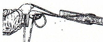
Рис. 1 «б». Закрепление спасательной веревки за конструкцию первым способом
