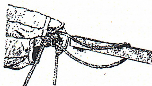
Рис. 1 «в». Закрепление спасательной веревки за конструкцию первым способом
